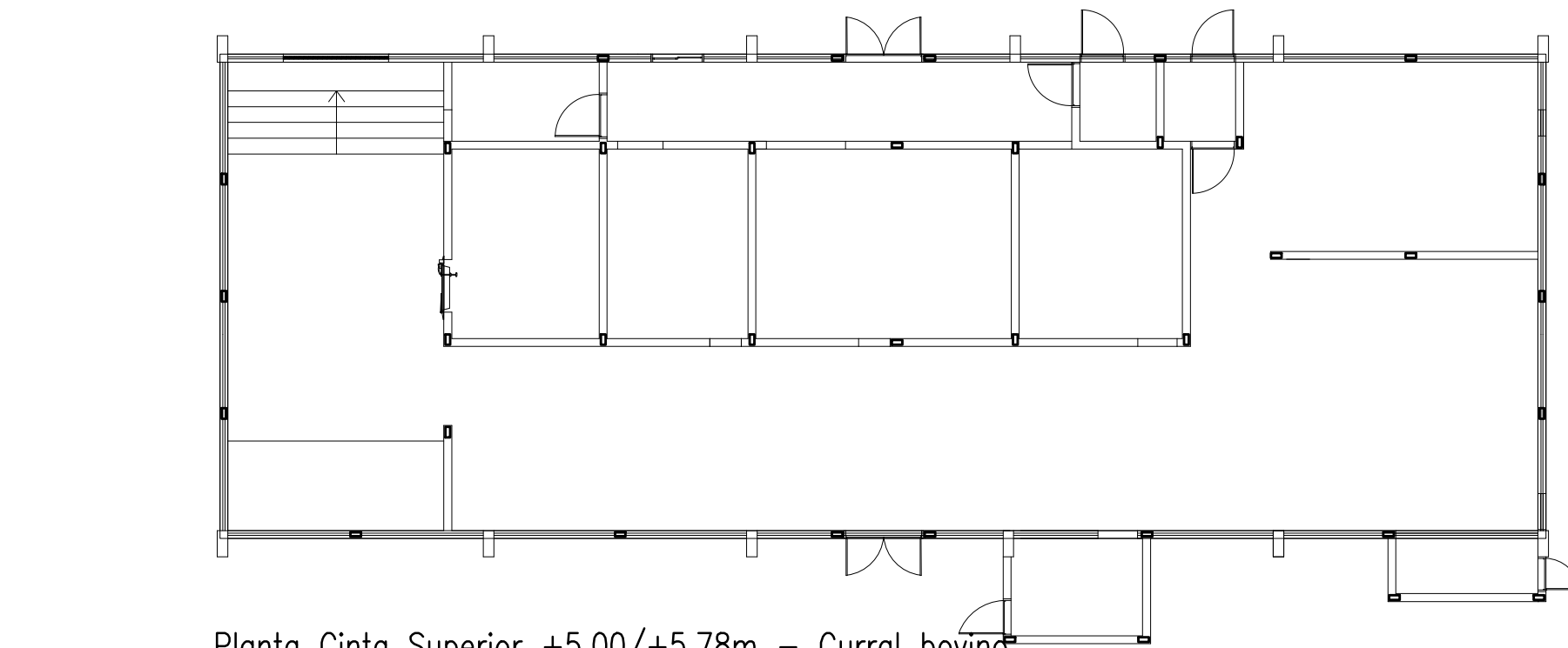
Planta Cinta Superior +5,00/+5,78m – Curral bovino escala + 1/125
