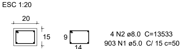
CINTA GERAL INFERIOR - CGI (PERÍMETRO: 135,33m)
